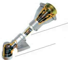
COPPIA CONICA CON 4 CUSCINETTI.
